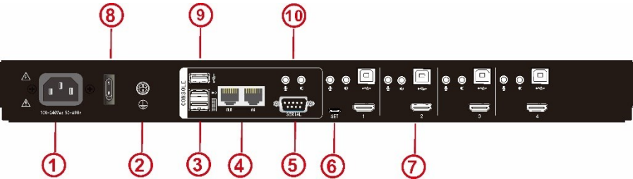
图 1.1 后视图
